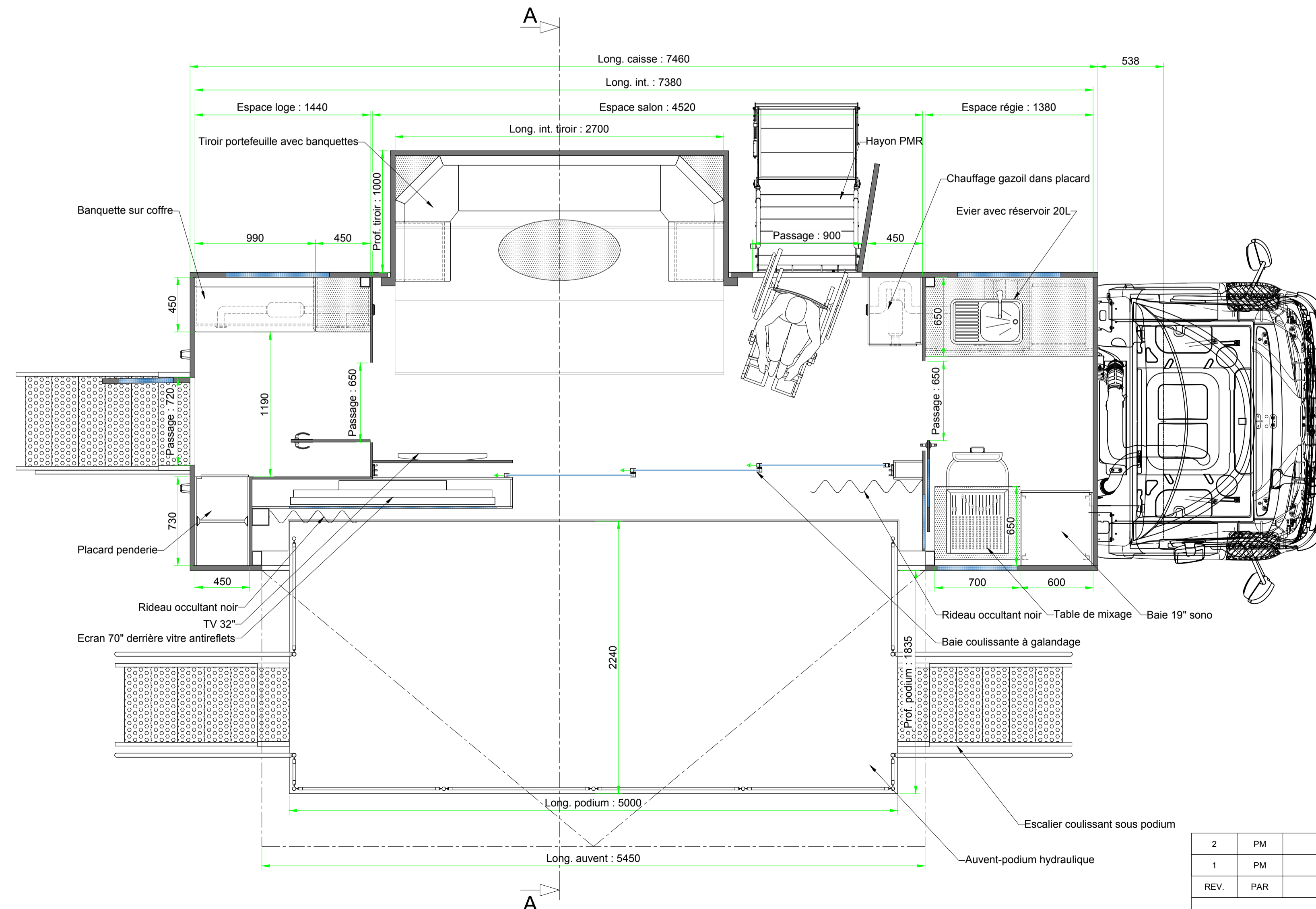
VUE DE DESSUS DE L'AMENAGEMENT
